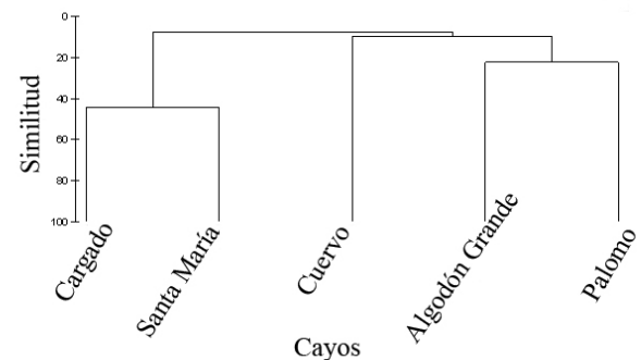
Figura 5. Análisis de conglomerados mostrando las relaciones entre los cayos Algodón Grande, Cargado, Cuervo, Palomo y Santa María sobre la base de los valores de similitud.
